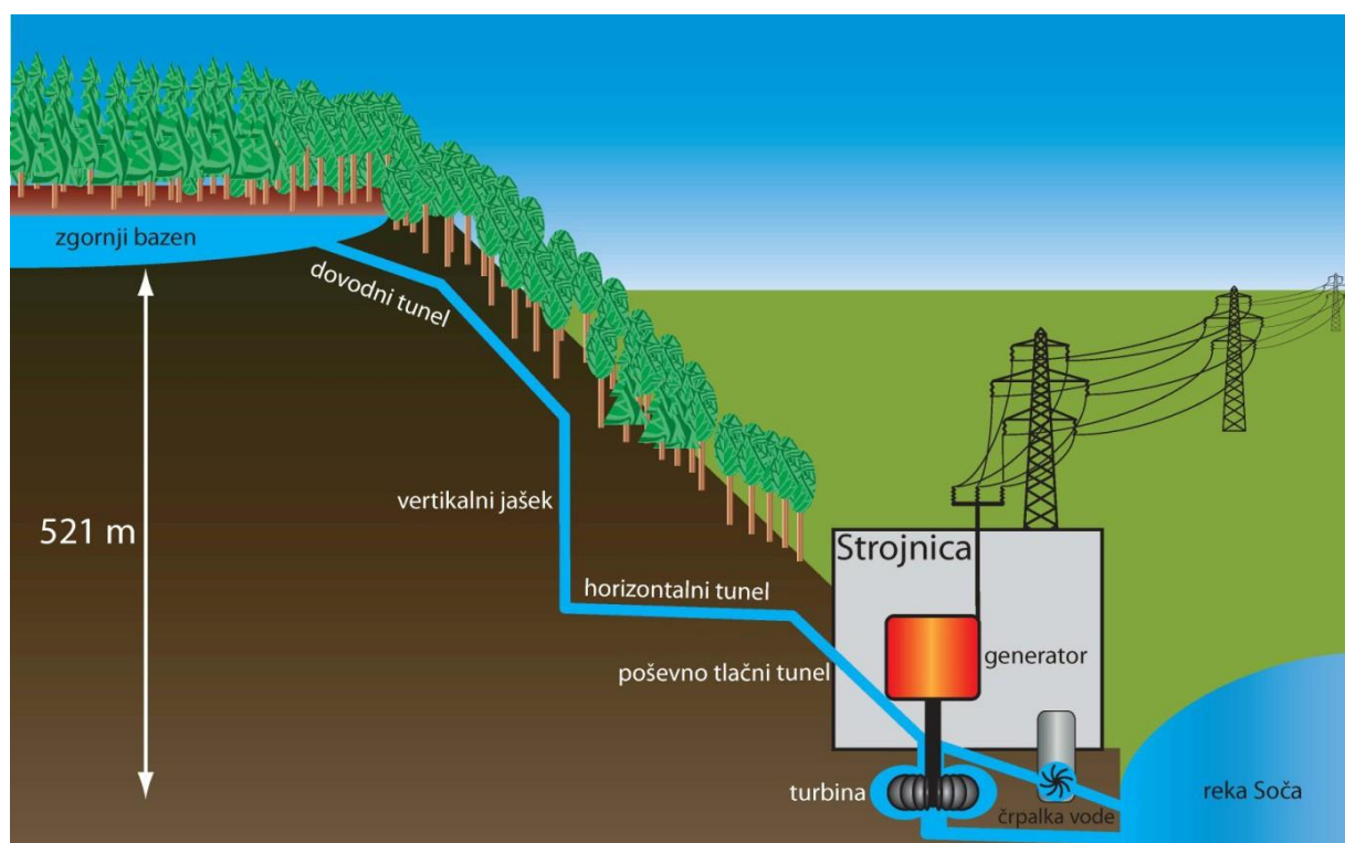
Na sliki: Prerez črpalne HE Avče
