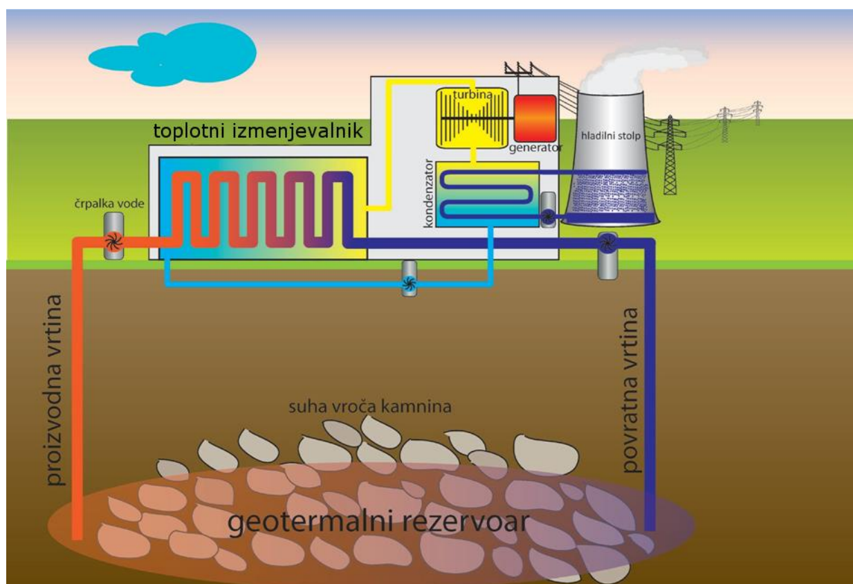
Na sliki: Tehnološka shema GE
